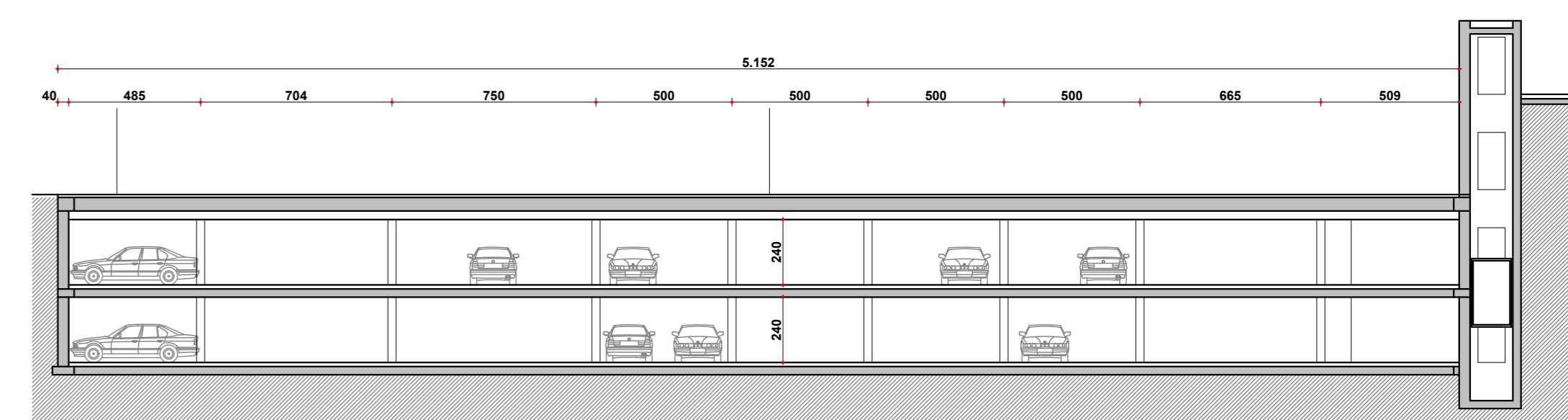
NUOVA AUTORIMESSA IN CESSIONE: sezione A-A - scala 1:200
