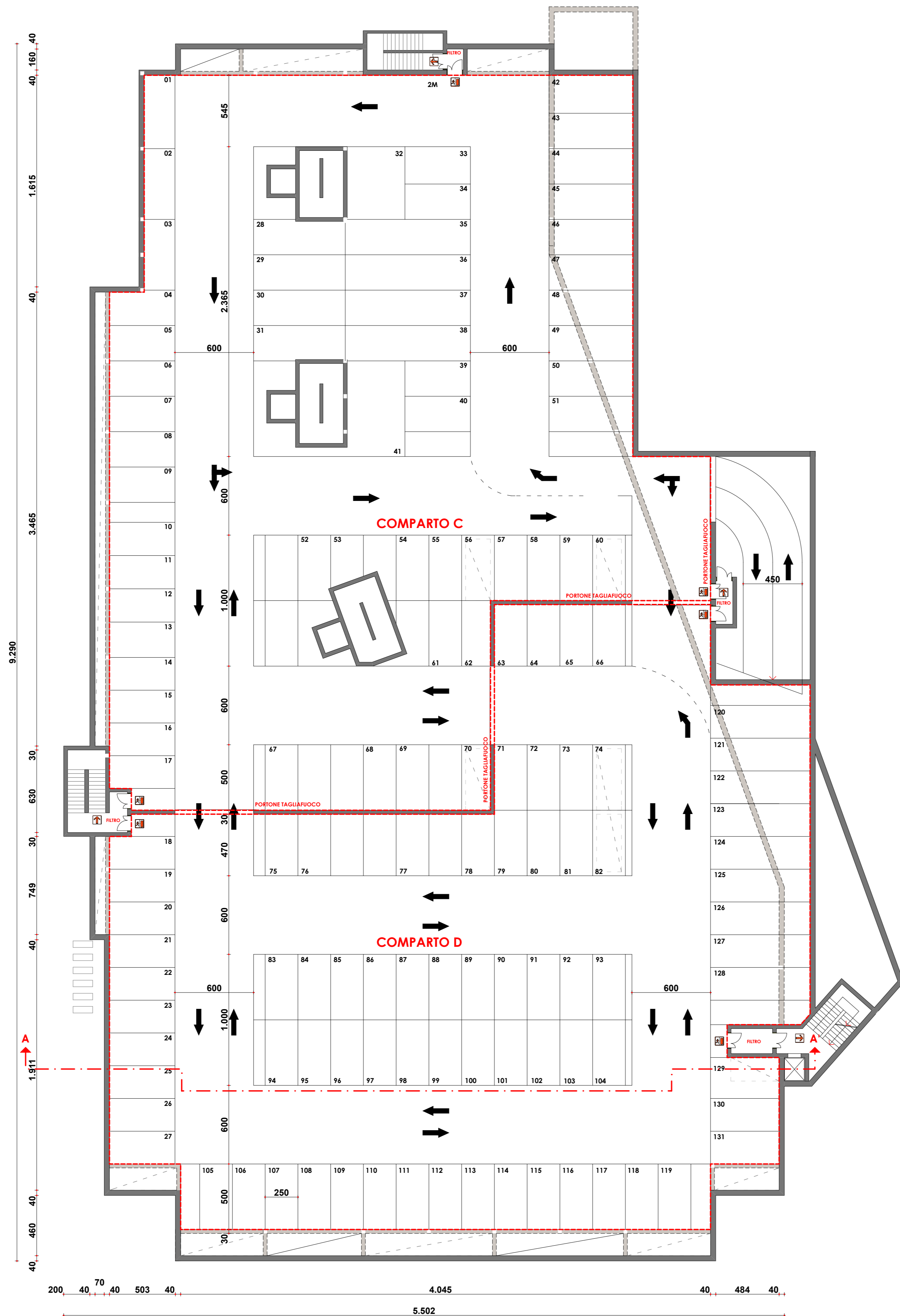
NUOVA AUTORIMESSA IN CESSIONE: pianta piano secondo interrato - scala 1:200
