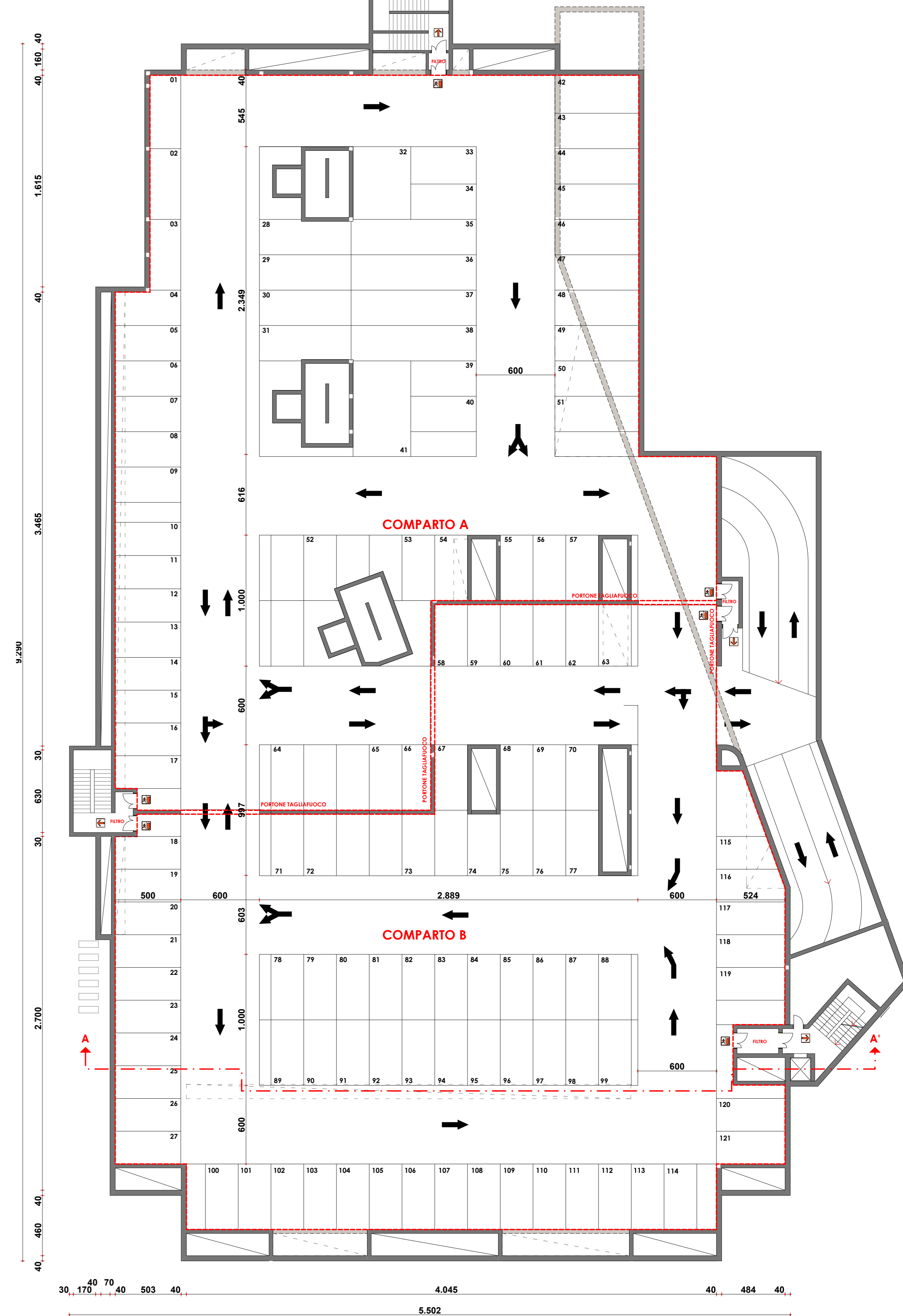
NUOVA AUTORIMESSA IN CESSIONE: pianta piano primo interrato - scala 1:200
