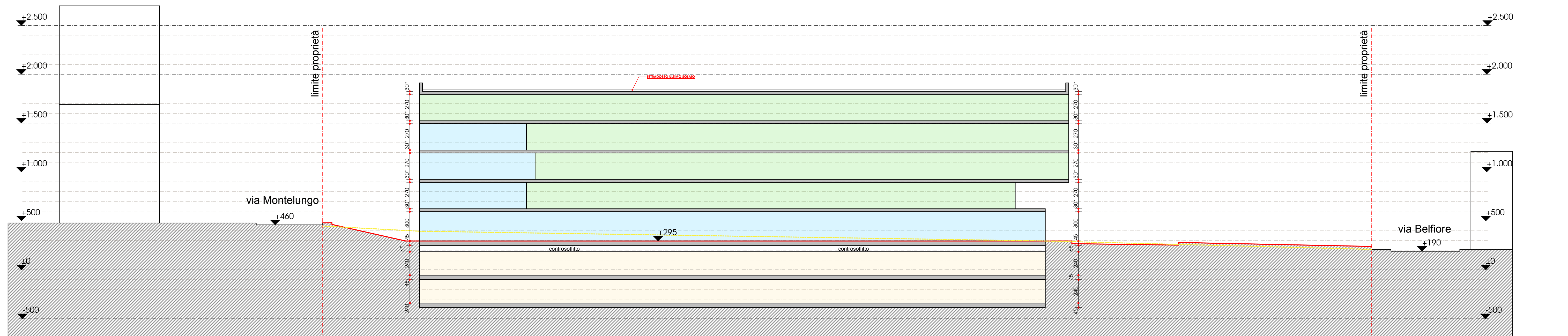
SEZIONE D/D' - scala 1:200
