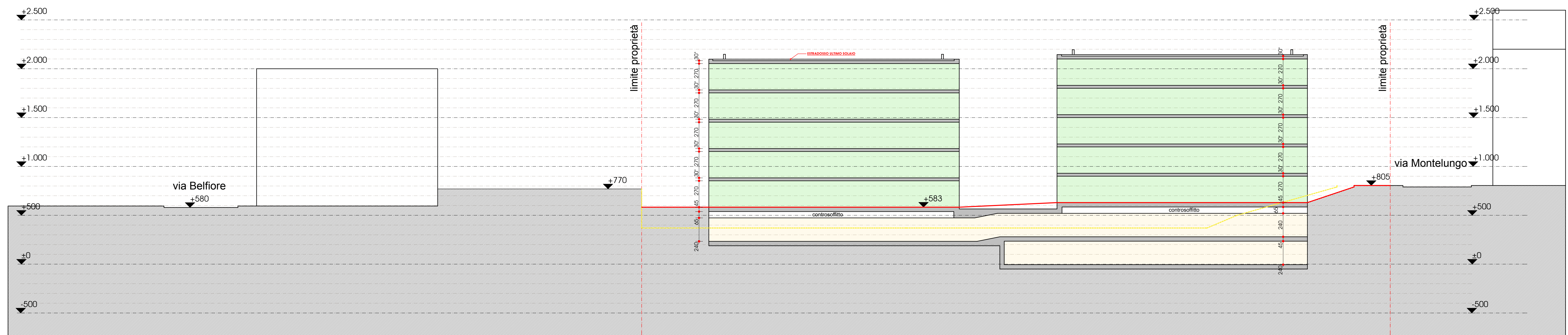
SEZIONE A/A' - scala 1:200
