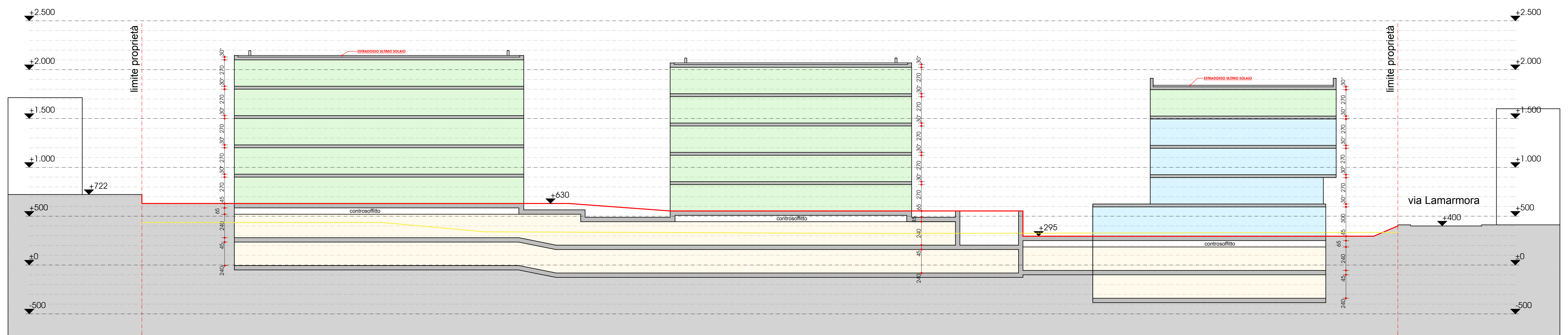
SEZIONE C/C' - scala 1:200
