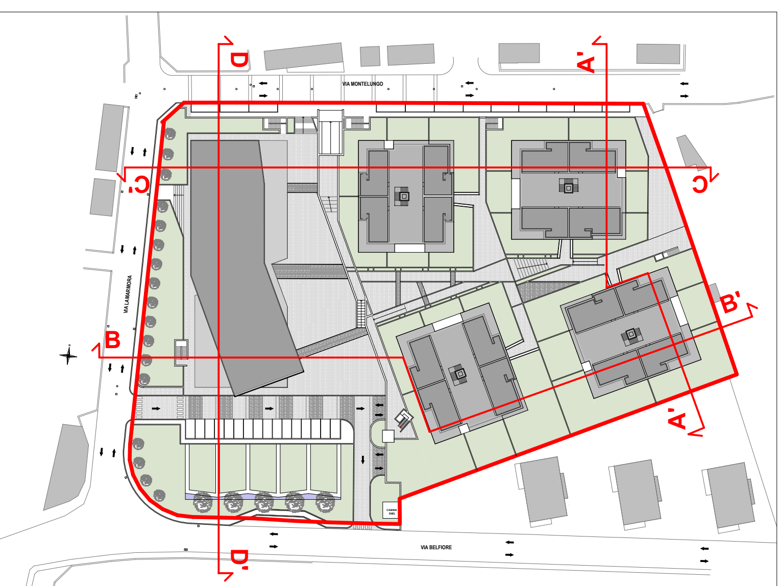
PLANIMETRIA - scala 1:1000 Unità minima di intervento
