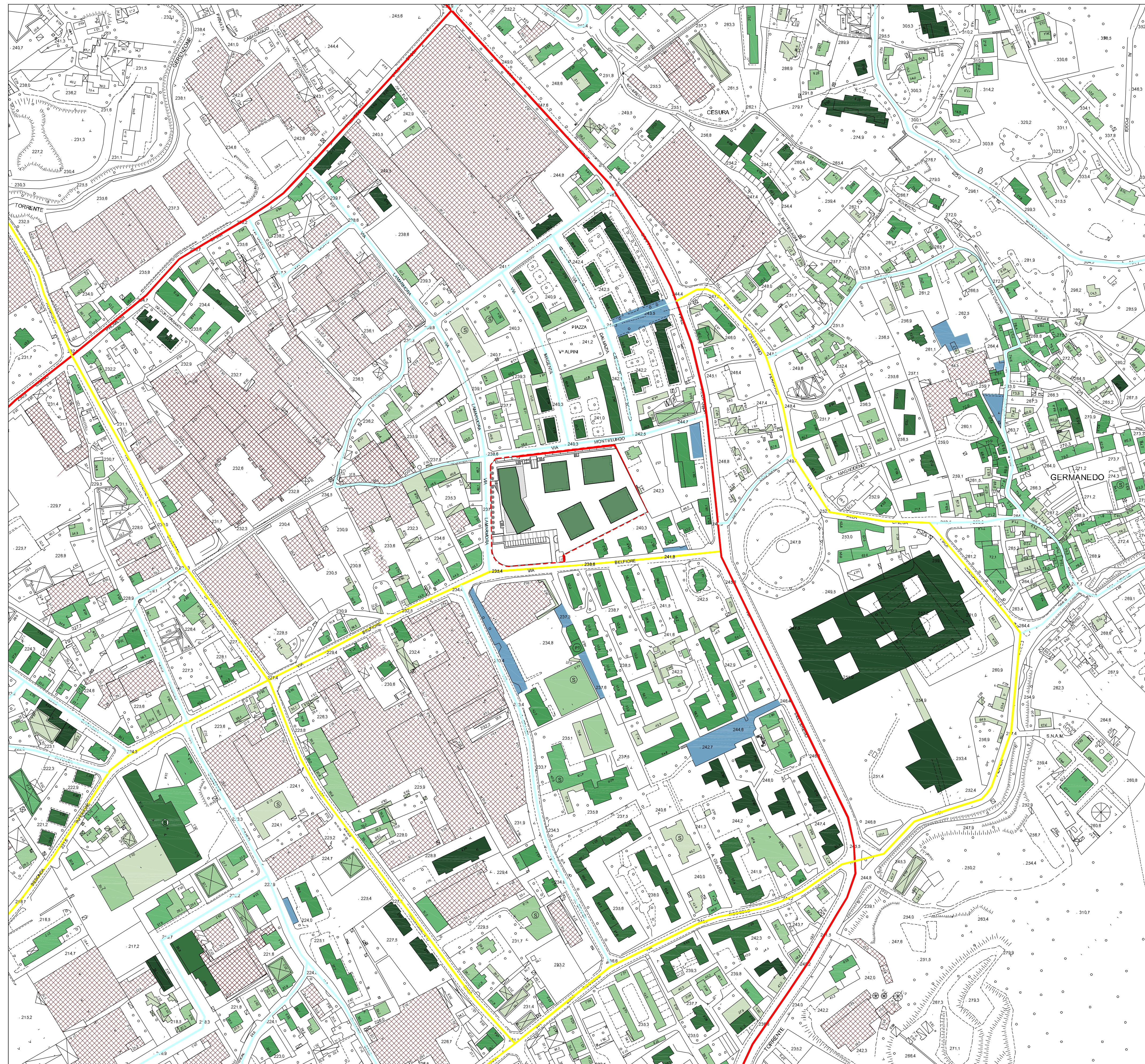
Viabilità e densità edilizia - scala 1:2000
